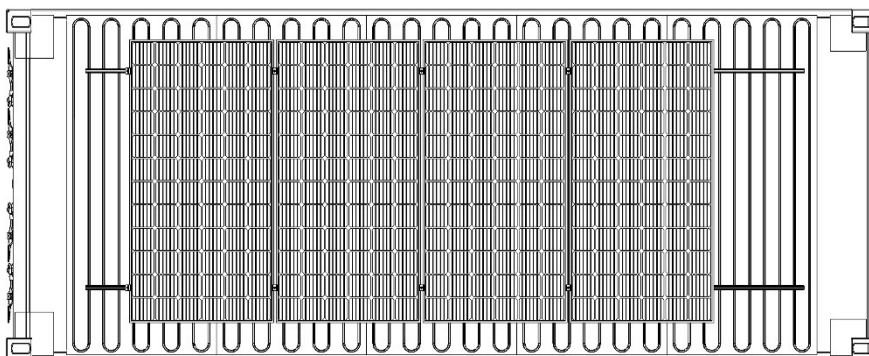
Rysunek 2: Widok poglądowy kontenera dach (góra). Propozycja systemu montażu paneli fotowoltaicznych z wykorzystania szyn montażowych.
